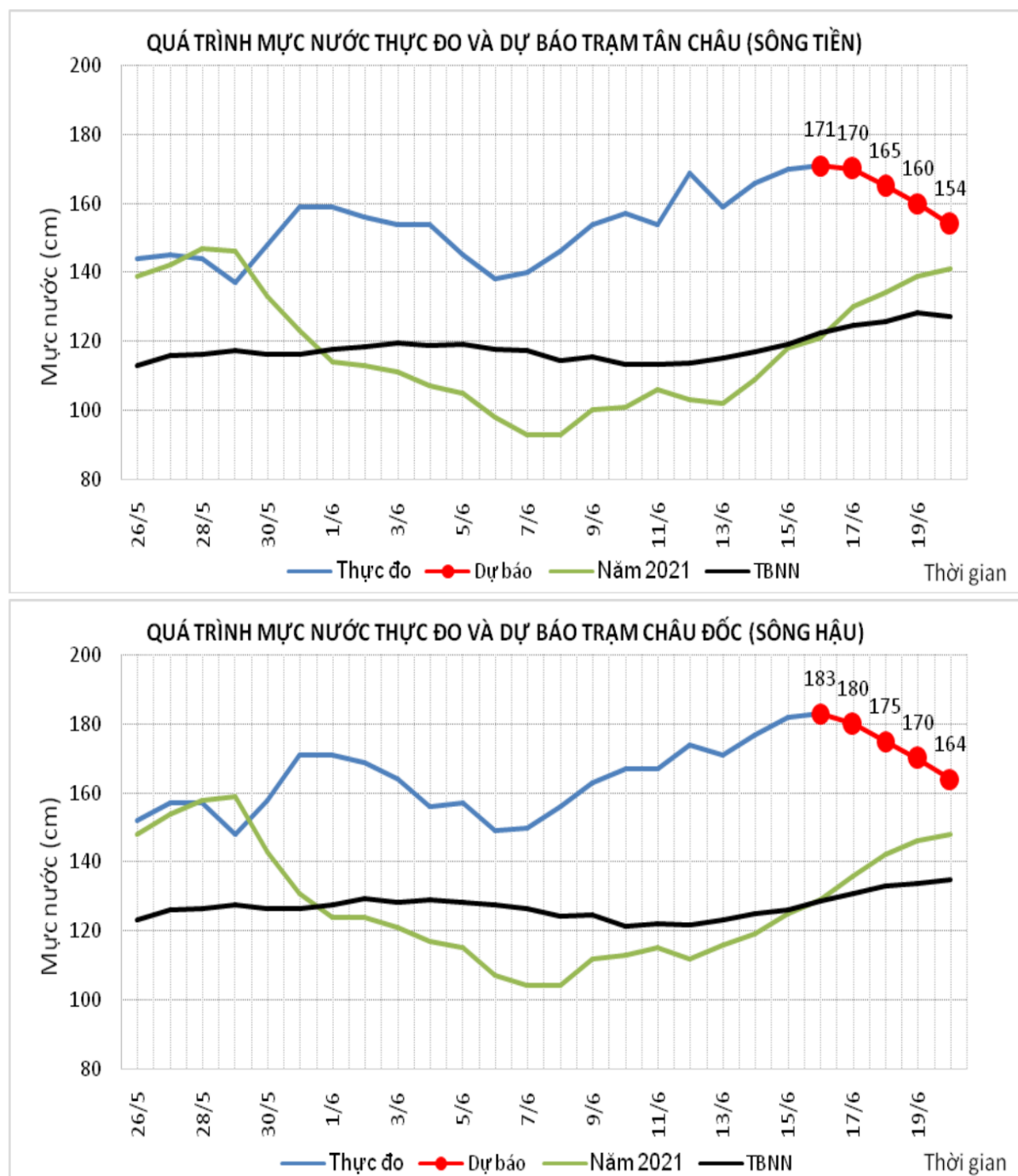
Hình 15. Đường quá trình mực nước thực đo và dự báo tại trạm Tân Châu và Châu Đốc từ 26/5 – 20/6/2022
