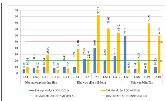
Hình 4. Biểu đồ TSS của vùng TGLX
