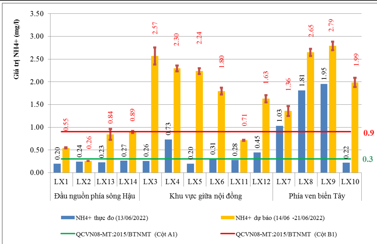
Hình 18. Biểu đồ giá trị NH_4^+ dự báo từ ngày 14/6 – 21/6/2022
