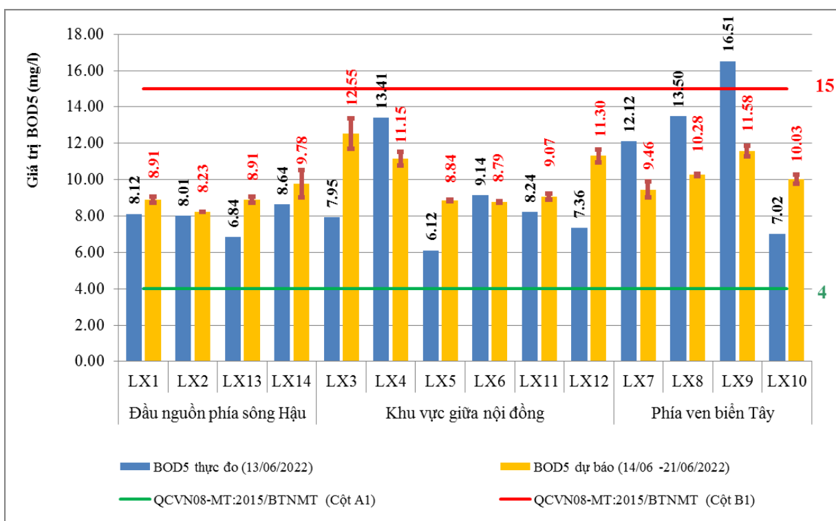
Hình 17. Biểu đồ giá trị BOD_5 dự báo từ ngày 14/6 – 21/6/2022
