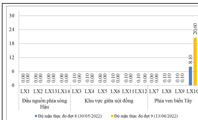
Hình 3. Biểu đồ độ mặn của vùng TGLX
