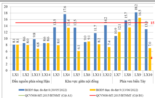
Hình 6. Biểu đồ BOD 5 của vùng TGLX
