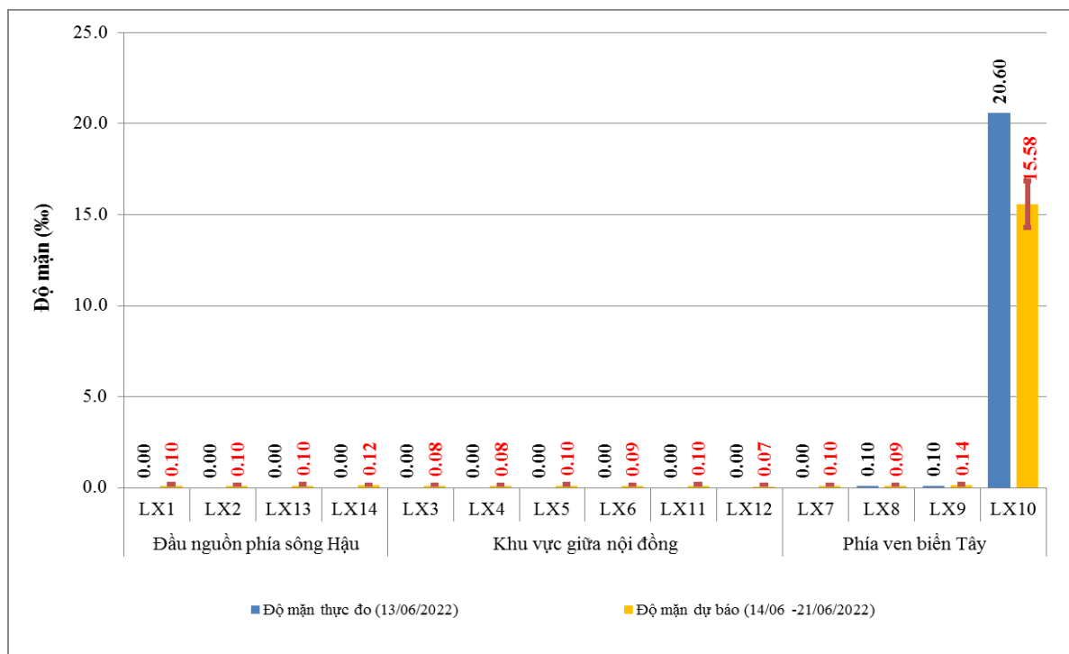
Hình 19. Biểu đồ giá trị độ mặn dự báo từ ngày 14/6 – 21/6/2022
