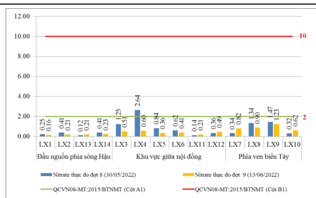
Hình 10. Biểu đồ NO_3^- của vùng TGLX
