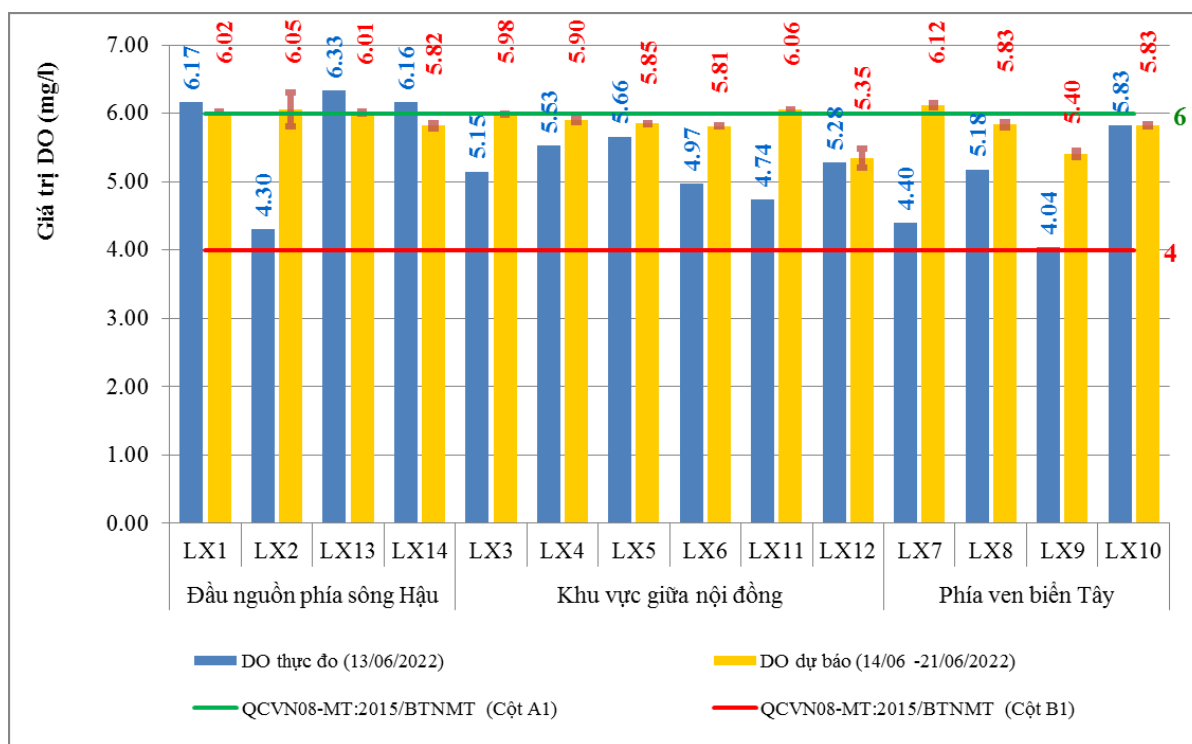
Hình 16. Biểu đồ giá trị DO dự báo từ ngày 14/6 – 21/6/2022
